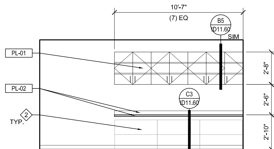
FILES 108 SCALE: 1/4"=1'-0"
